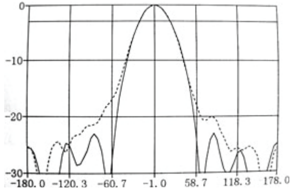
4000MHz(43° /43° )
