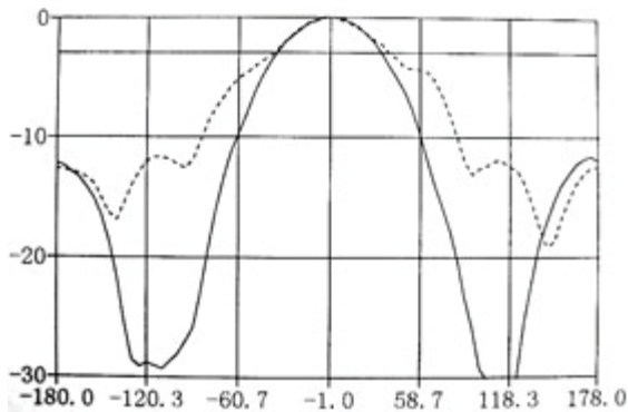
2000MHz(76° /68° )
