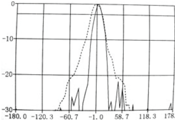
16000MHz(24° /15° )
