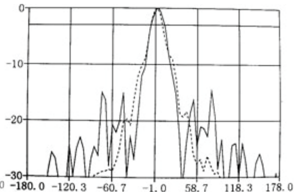
18000MHz(16° /19° )
