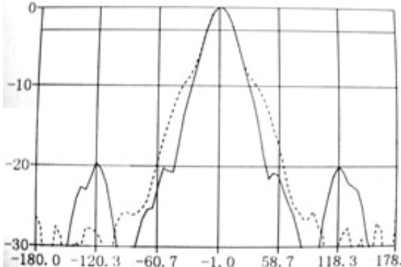
8000MHz(27° /27° )
